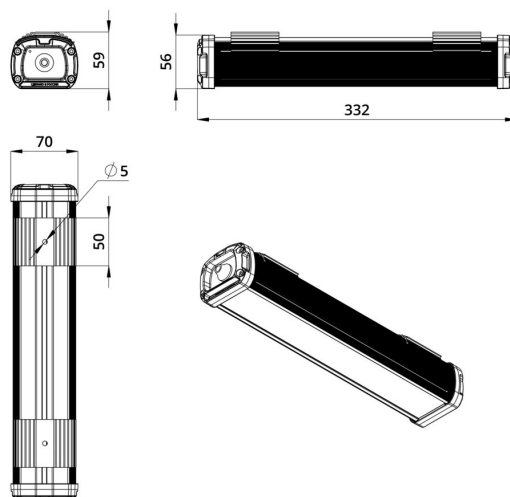
Габаритный чертеж
