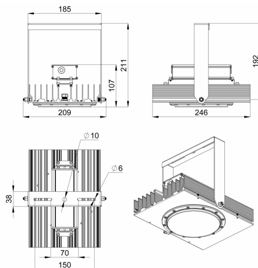
Габаритный чертеж
