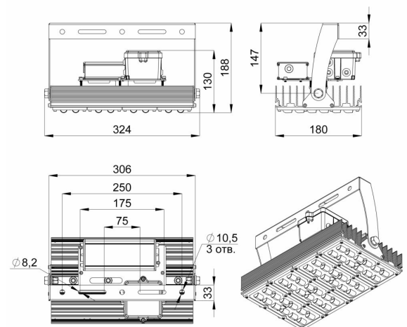
Габаритный чертеж
