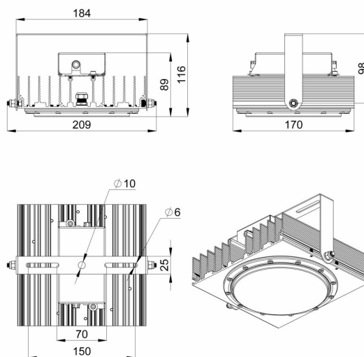
Габаритный чертеж
