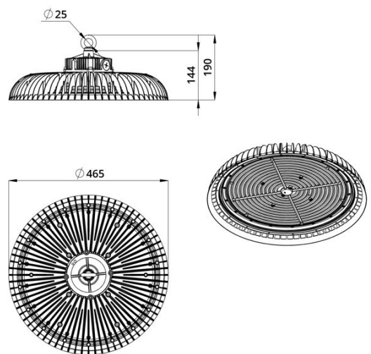
Габаритный чертеж
