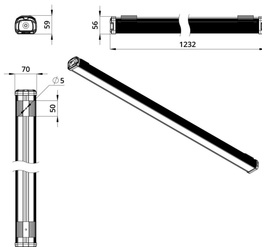
Габаритный чертеж
