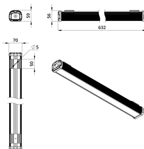
Габаритный чертеж
