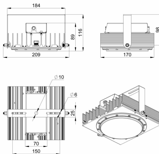
Габаритный чертеж
