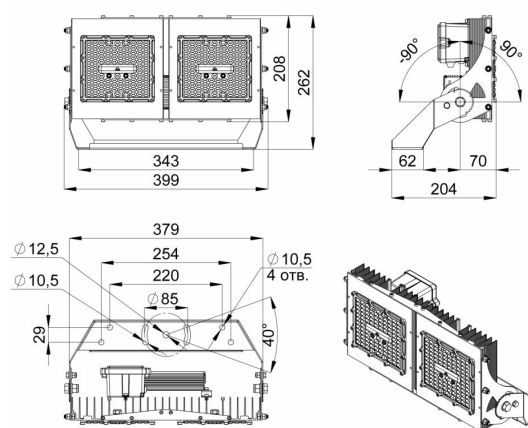
Габаритный чертеж
