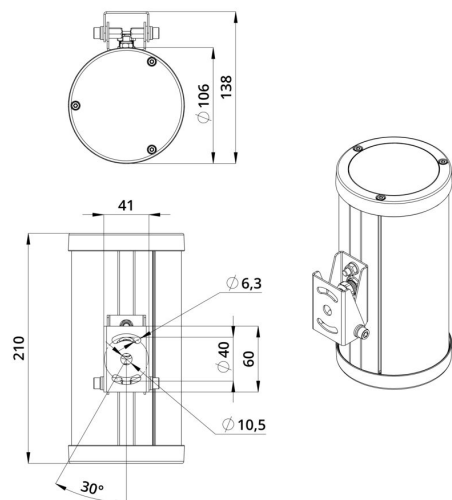
Габаритный чертеж
