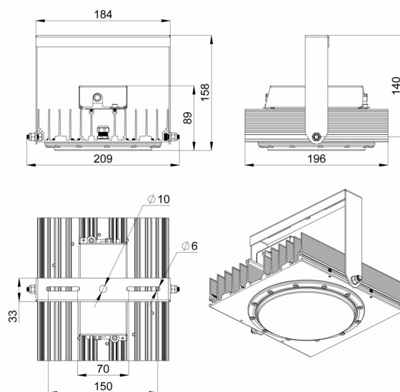
Габаритный чертеж
