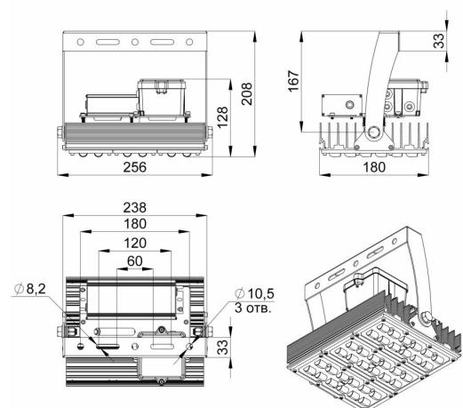
Габаритный чертеж
