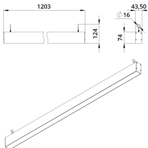
Габаритный чертеж
