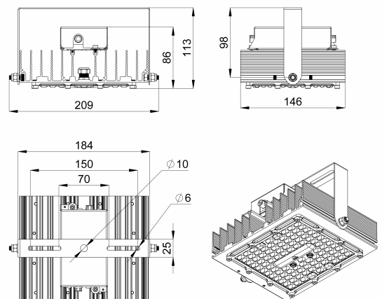
Габаритный чертеж
