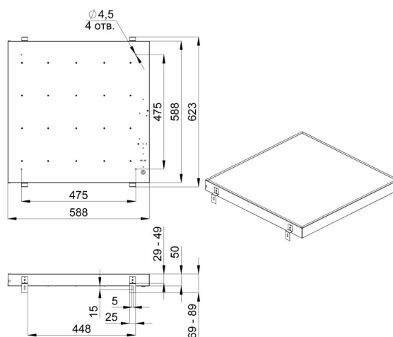
Габаритный чертеж
