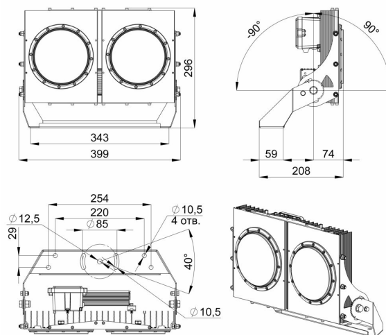
Габаритный чертеж
