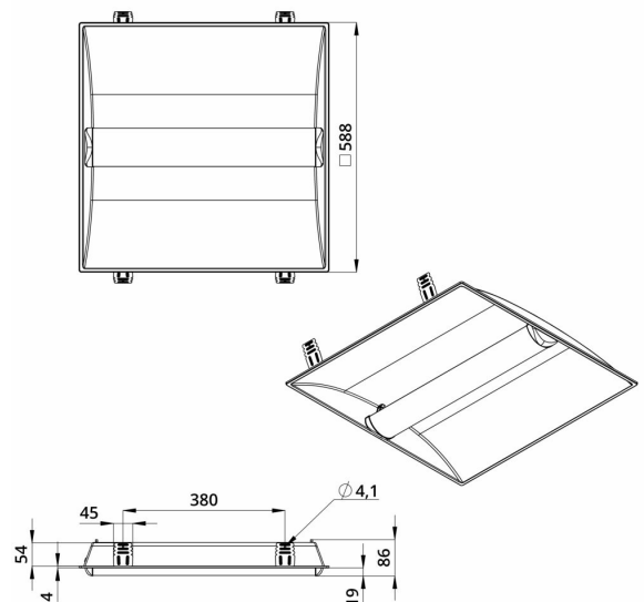
Габаритный чертеж
