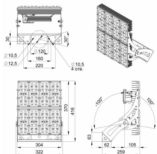
Габаритный чертеж
