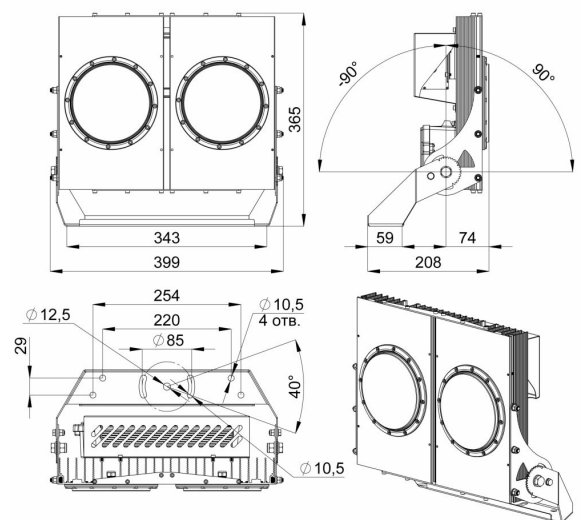
Габаритный чертеж
