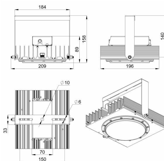
Габаритный чертеж
