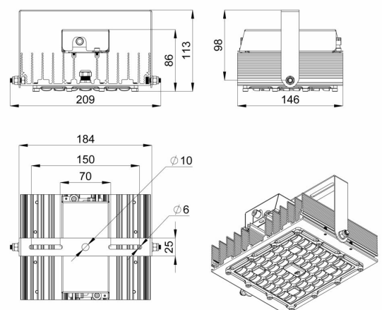
Габаритный чертеж
