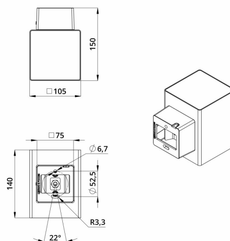
Габаритный чертеж
