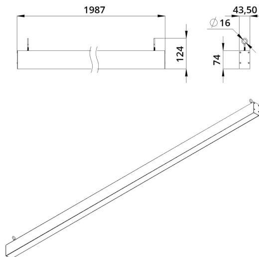
Габаритный чертеж
