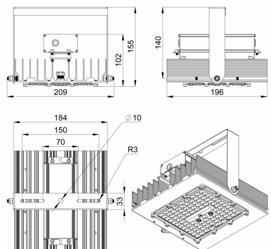
Габаритный чертеж
