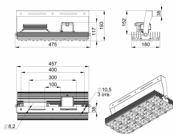
Габаритный чертеж
