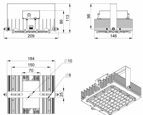
Габаритный чертеж
