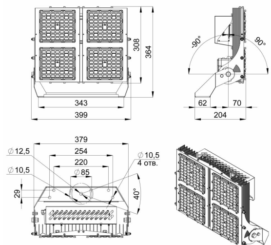
Габаритный чертеж
