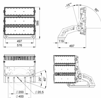
Габаритный чертеж
