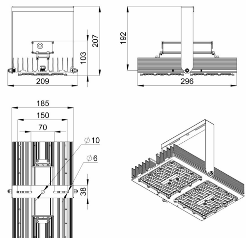
Габаритный чертеж
