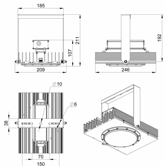
Габаритный чертеж
