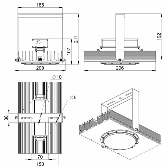
Габаритный чертеж
