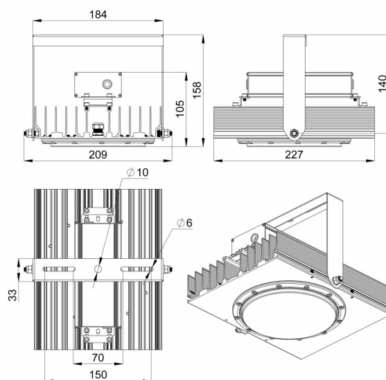
Габаритный чертеж
