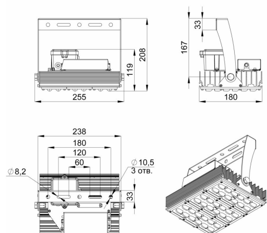
Габаритный чертеж
