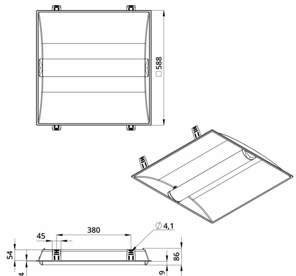
Габаритный чертеж
