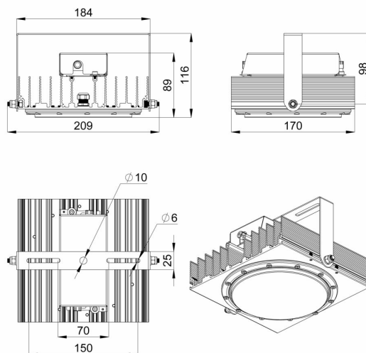
Габаритный чертеж
