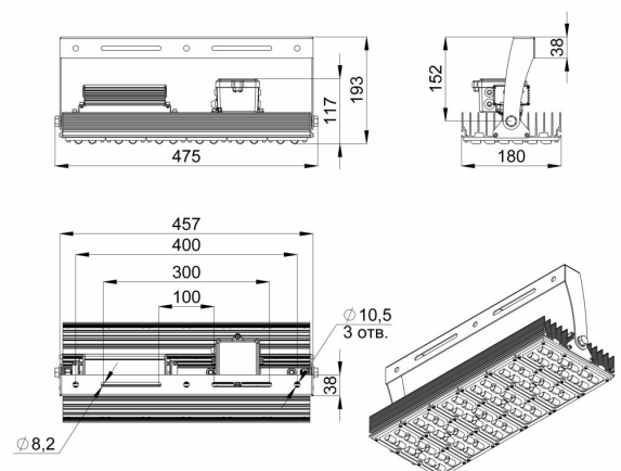
Габаритный чертеж
