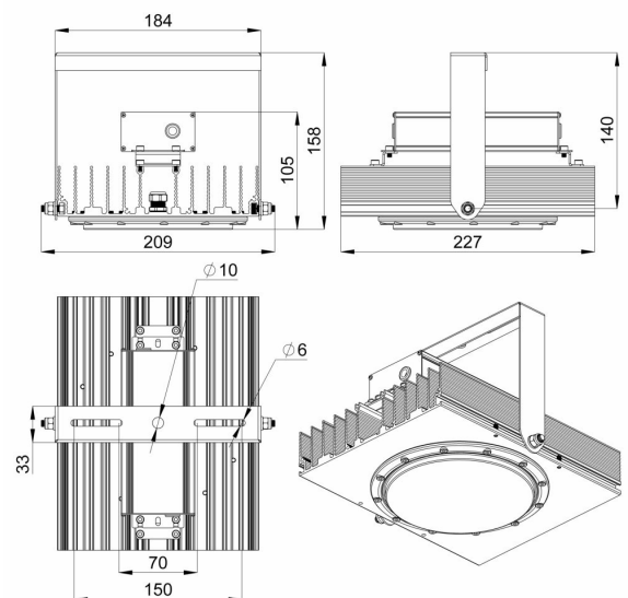
Габаритный чертеж
