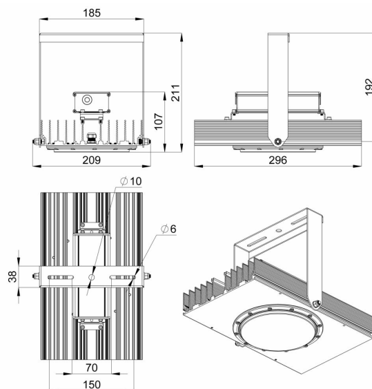
Габаритный чертеж
