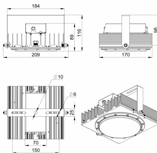
Габаритный чертеж
