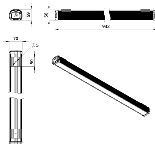
Габаритный чертеж
