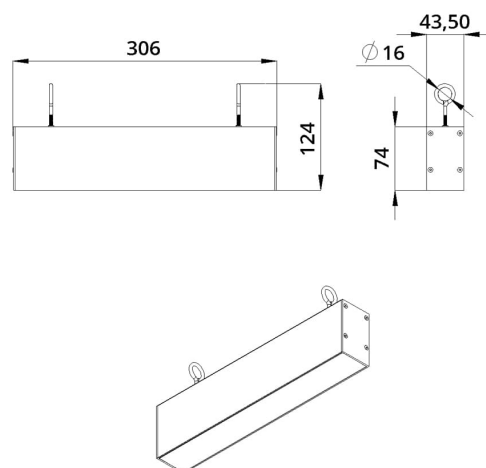
Габаритный чертеж
