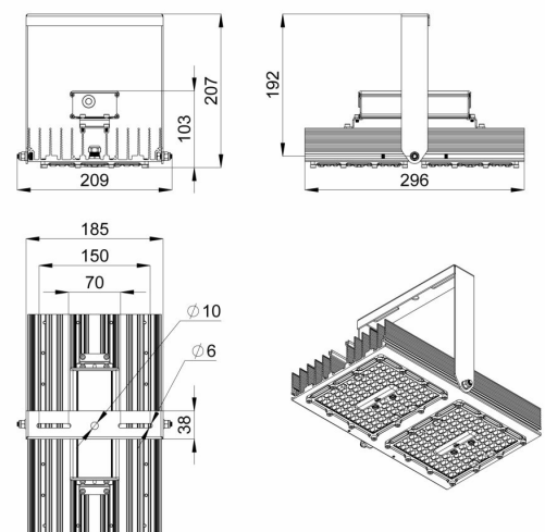
Габаритный чертеж
