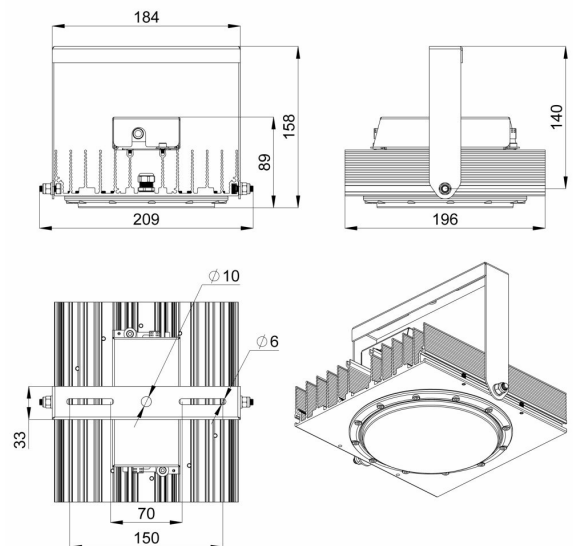
Габаритный чертеж
