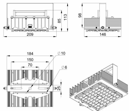
Габаритный чертеж
