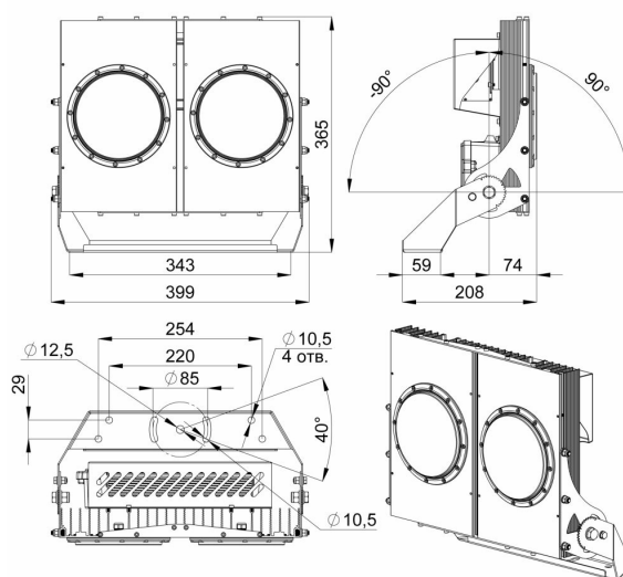
Габаритный чертеж
