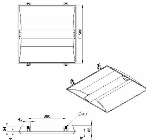
Габаритный чертеж
