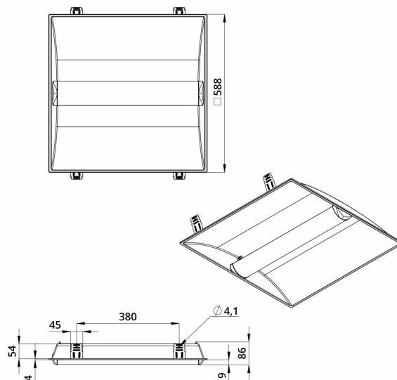
Габаритный чертеж
