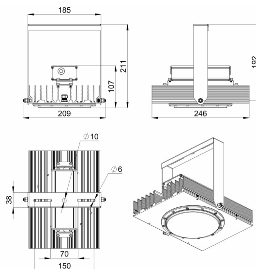
Габаритный чертеж
