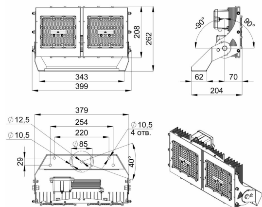
Габаритный чертеж
