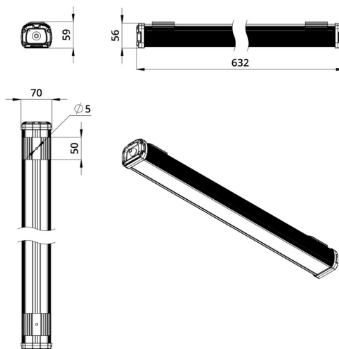
Габаритный чертеж
